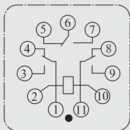
图 2 底视接线图(JQX-10F/3Z)
