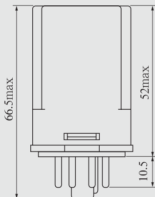
图 3 外形图(JQX-10F/2Z)
