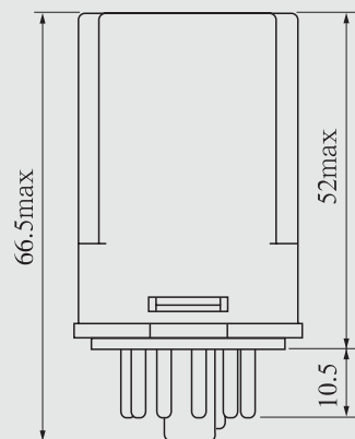
图 4 外形图(JQX-10F/3Z)
