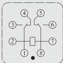
图 1 底视接线图(JQX-10F/2Z)
