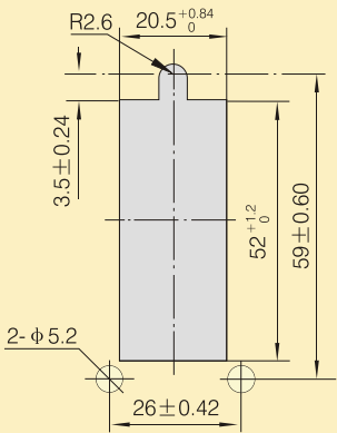
DZ-60屏面开孔图
