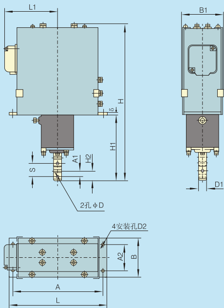
MZS1-25H、45H、80H电磁铁外形及安装尺寸
