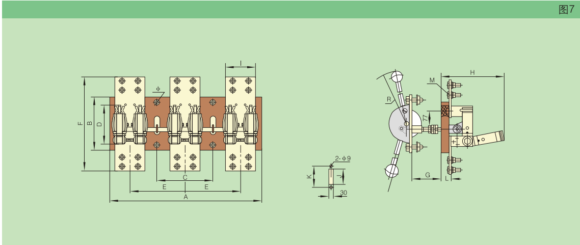
4.7 HD13外形及安装尺寸(见图7、表8)
