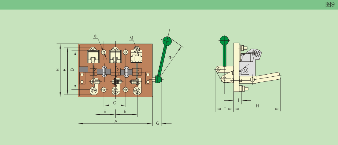
4.9 HD14外形及安装尺寸(见图9、表10)
