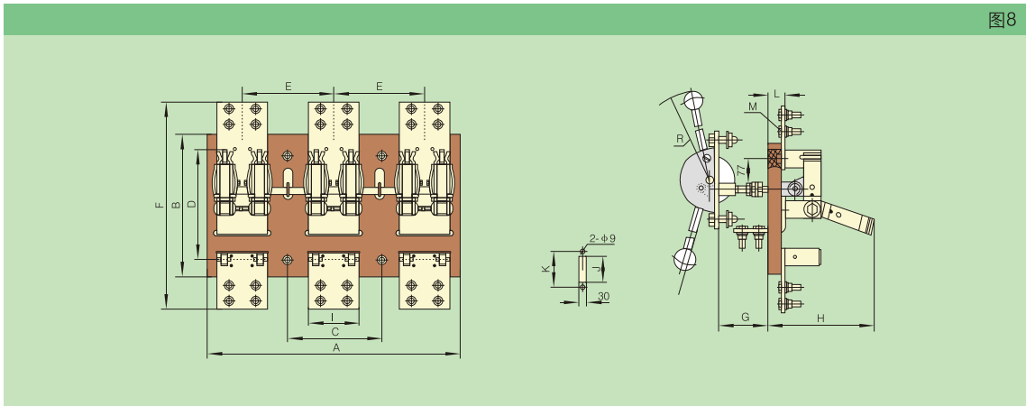
4.8 HS13外形及安装尺寸(见图8、表9)
