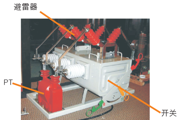
适用于配电自动化的组合开关
