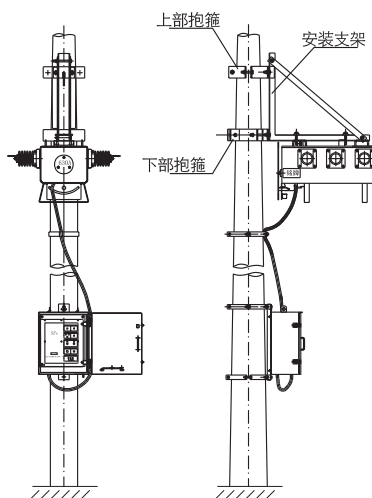
吊装布置示意图
