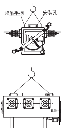
起吊示意图
