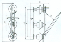
GW1-6、10/200、400、630型外形尺寸
