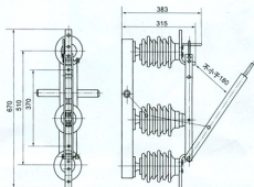
GW1-10W/200、400、630型外形尺寸
