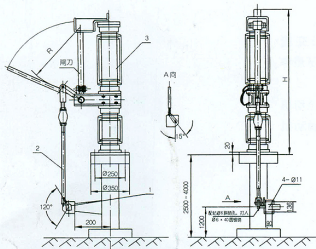
GW8-35、60、110(W)/400型中性点隔离开关
