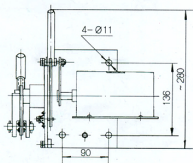
CS8-1型手力操动机构外形尺寸图
