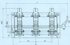
GN6-6T/200-1, 400-1 GN6-10T/200-1, 400-1, 630-1, 1250-1 型外形尺寸图 (II、III型的高和安装尺寸与I型相同)
