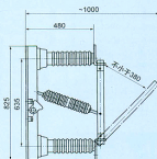
GN6-6T/200-1, 400-1 GN6-10T/200-1, 400-1, 630-1, 1250-1 型外形尺寸图 (II、III型的高和安装尺寸与I型相同)
