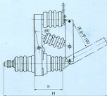
GN6-6T/200-1, 400-1 GN6-10T/200-1, 400-1, 630-1, 1250-1 型外形尺寸图 (II、III型的高和安装尺寸与I型相同)
