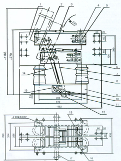
GN10-20/8000、10000型户内隔离开关外形图
