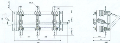
GN19-10/400、630型外形尺寸图
