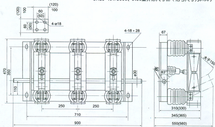
GN25-10T/2000、3150型外形尺寸图 (括号尺寸为3150)
