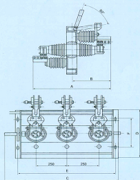
GN30-10D/2000、2500、3150型外形尺寸图
