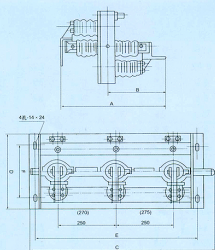
GN30-10/400、630、1000、1250型外形尺寸图
