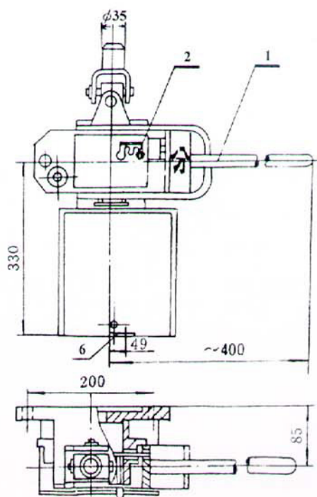
G5 水平操作—带辅助开关、接线板
