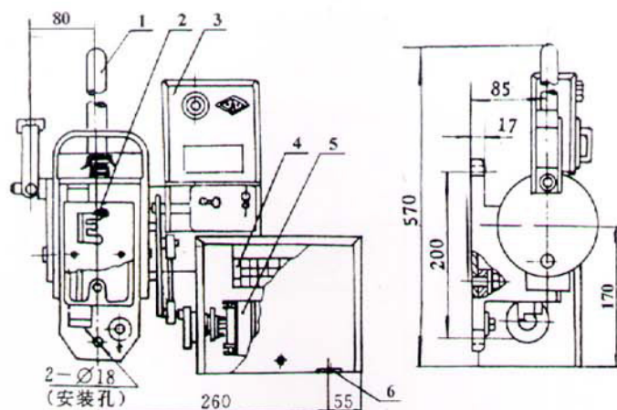
G1 竖直操作—带电磁锁、接线板、辅助开关
