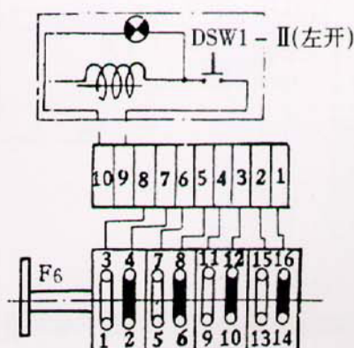
G1、G2 合闸时配线图
