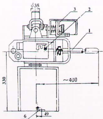
G5 水平操作—附装挂编码锁装置
