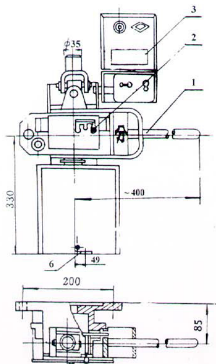
G4 水平操作—带电磁锁、接线板、辅助开关
