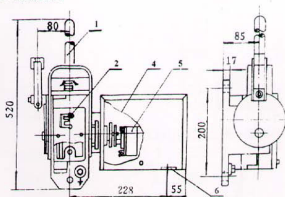
G2 竖直操作—附装挂编码锁装置
