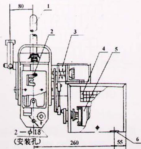
G2 竖直操作—带辅助开关、接线板
