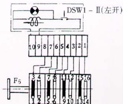
G1、G2 合闸时配线图
