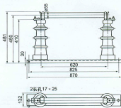
RN2-35/0.5型外形尺寸
