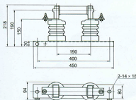
RN2-3、6、10/0.5型外形尺寸
