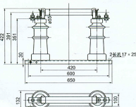
RN2-15、20/0.5型外形尺寸
