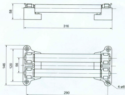
RNZ1 型双管外形尺寸
