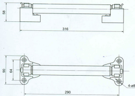
RNZ 型单管外形尺寸
