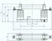
RN5-3、6、10/2-20型外形尺寸
