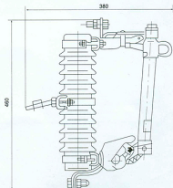
RW11-12 型外形尺寸
