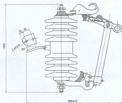
RW3-12 型外形尺寸
