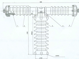
RW10-35型外形尺寸
