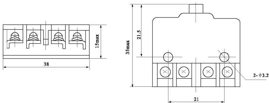
LX19K 外形及安装尺寸
