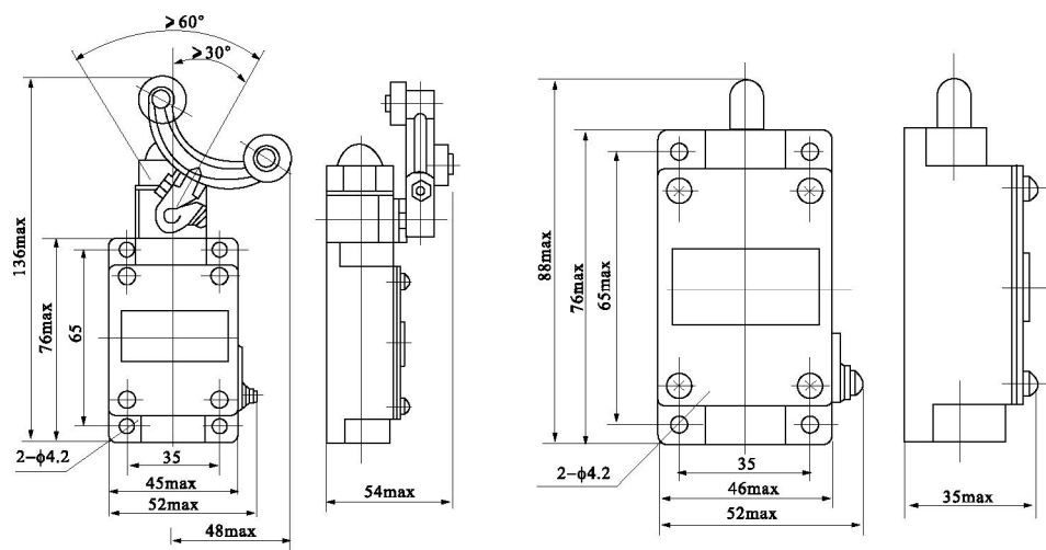
LX19-212、222、232 外形及安装尺寸
