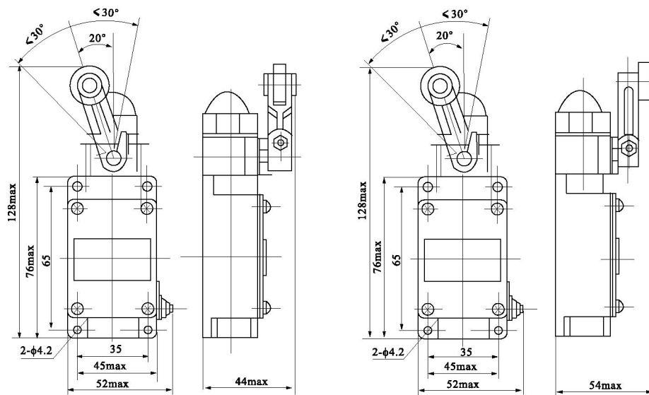
LX19-131 外形及安装尺寸
