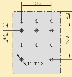
PCB安装孔位图(3Z)
