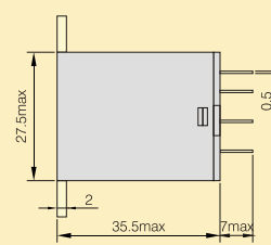
顶法兰式左视图
