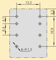
PCB安装孔位图(2Z)
