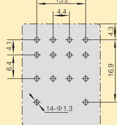
PCB安装孔位图(4Z)
