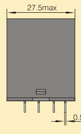
PCB式左视图
