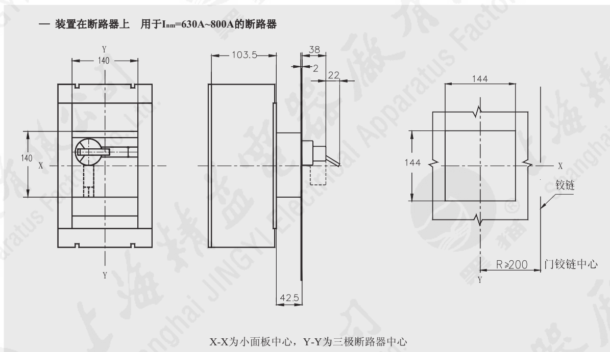
图 3-6 CS2-630、800转动手柄操作机构
