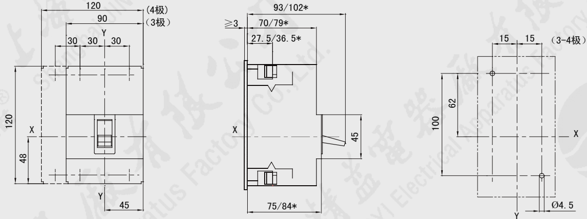
板前接线（热磁式）
