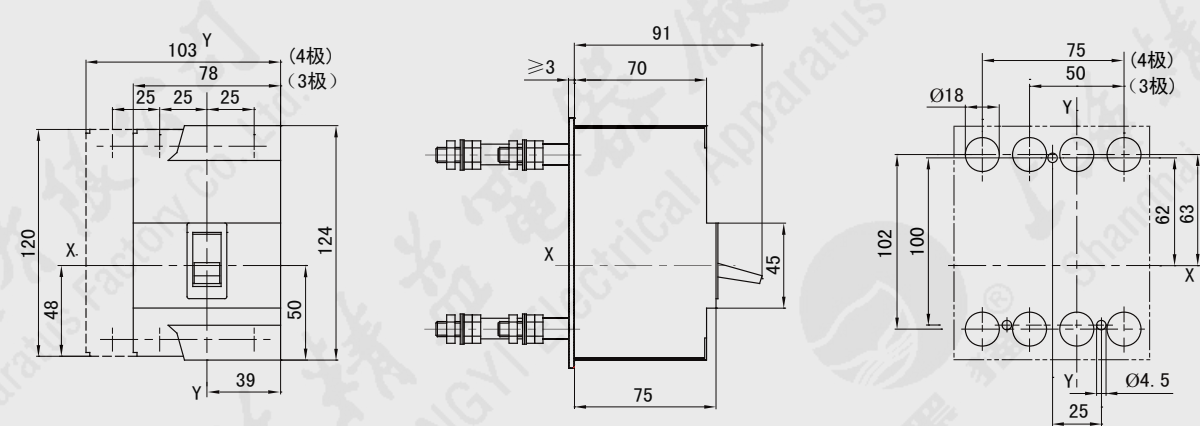
板后螺杆接线（热磁式）
