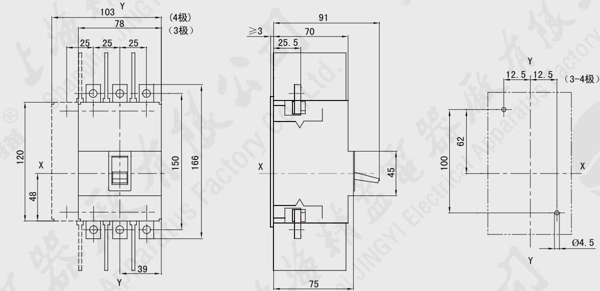
加长板前接线（热磁式）
