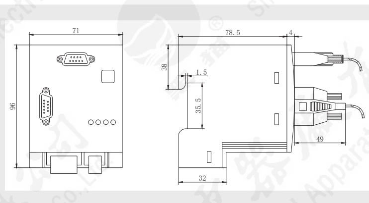
图2-12 ST-DP型通讯协议模块外形及安装尺寸图
