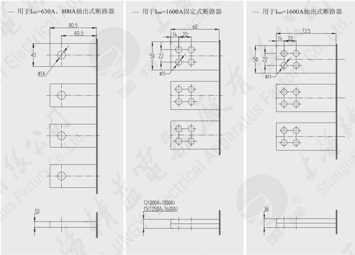
图 3-2 I nm =630A~1600A的断路器-板后水平接线，板后垂直接线
