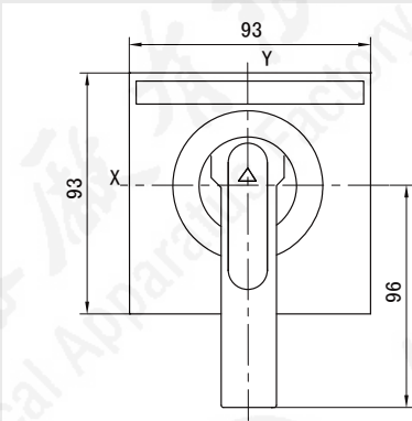
F-2 型 (用于HM3-630A~800A)
