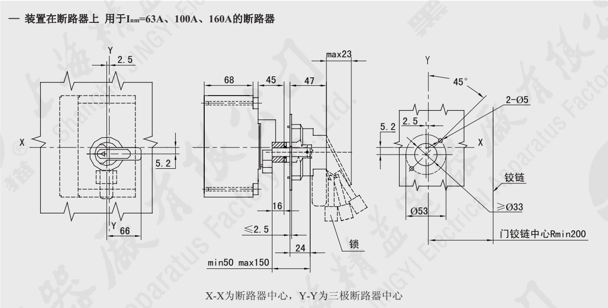
图 3-11 CS3-100、160转动手柄操作机构(偏心式)
