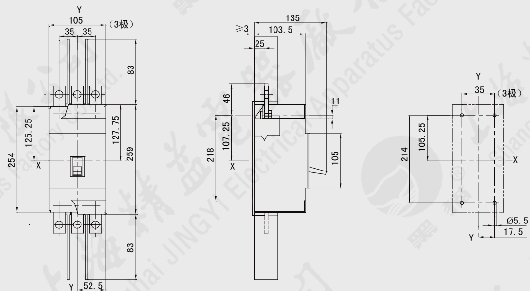
加长板前接线（电子式）
