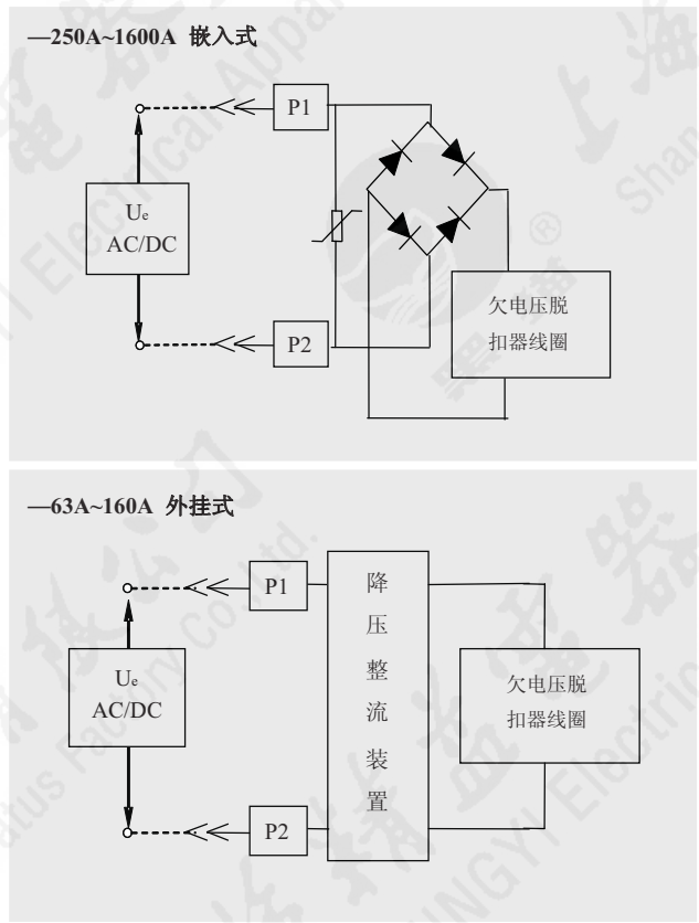
图 3-15 欠电压脱扣器二次回路接线图
