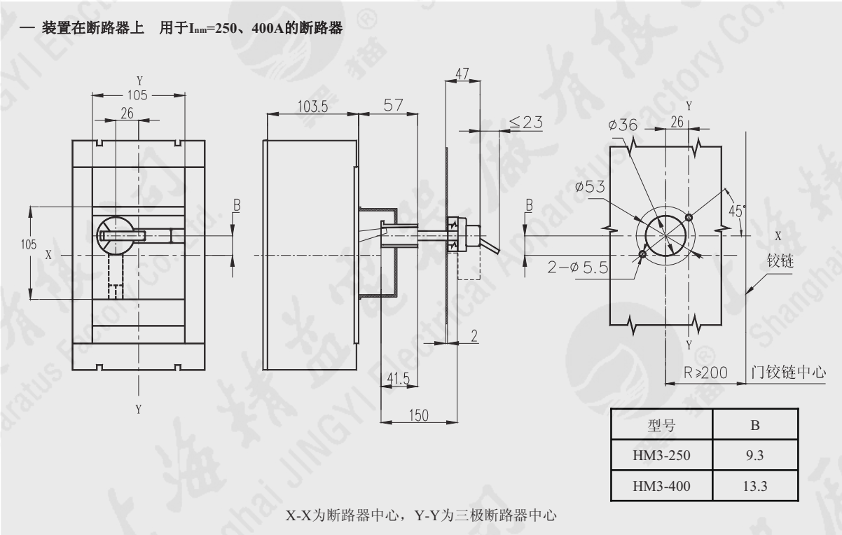
图 3-12 CS3-250、400转动手柄操作机构(偏心式)
