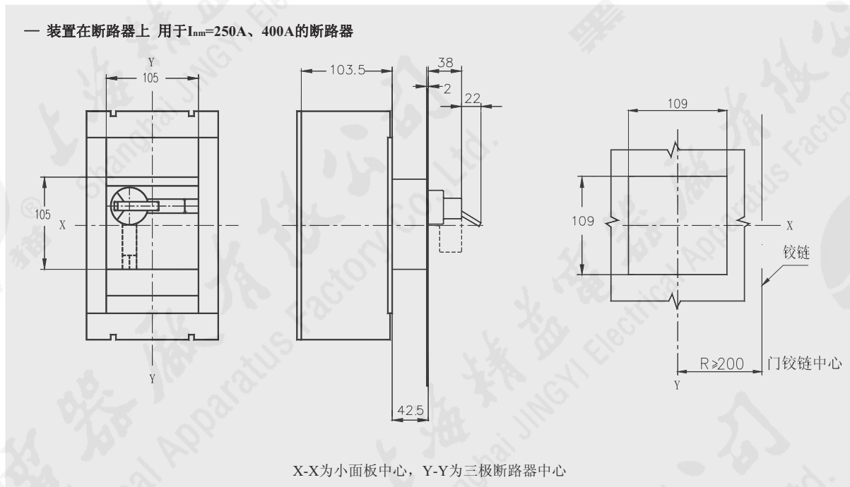
图 3-5 CS2-250、400转动手柄操作机构
