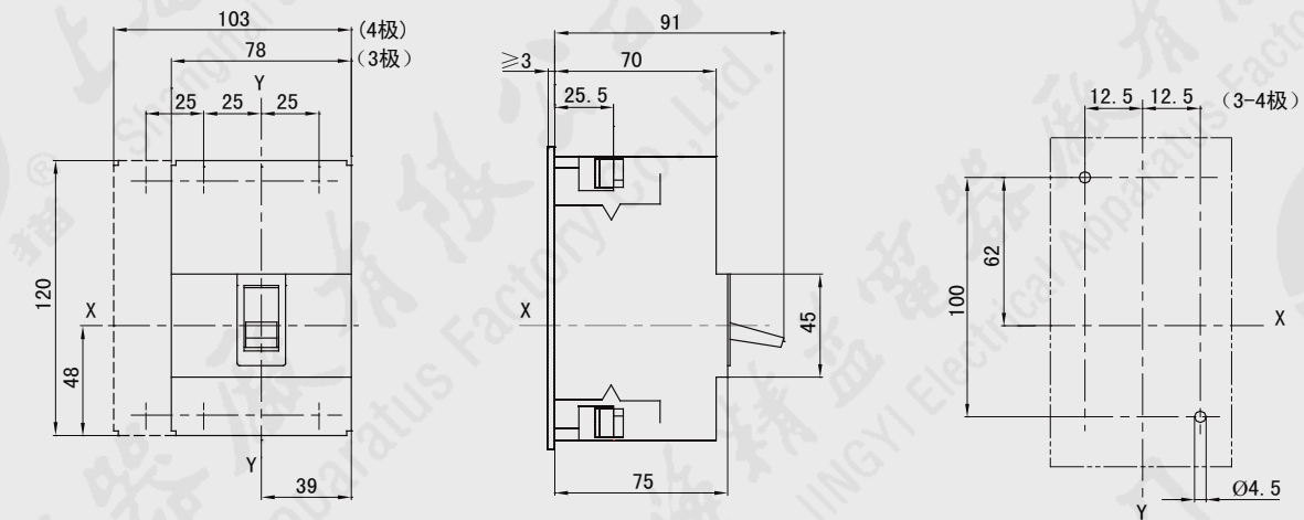
板前接线（热磁式）
