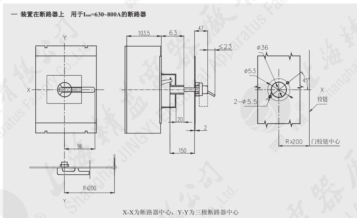
图 3-10 CS1-630、800转动手柄操作机构(中心式)
