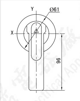
A-2 型 (用于HM3-630A~800A)
