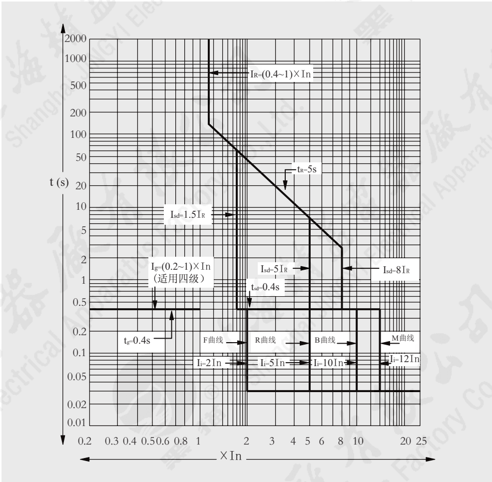
图 2-5 ST110-M 电子式脱扣器保护特性曲线( I^2t OFF)
