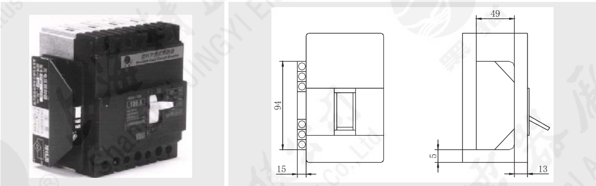
图1-15 63-160A外挂式欠电压脱扣器外形及安装尺寸
