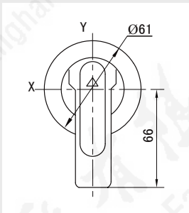
A-1 型 (用于HM3-63A~400A)
