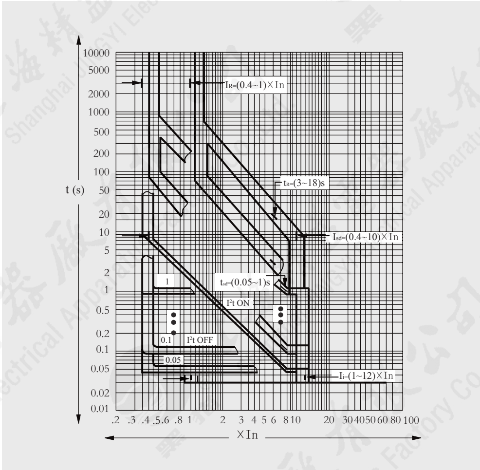
图 2-6 ST110-H 电子式脱扣器保护特性曲线
