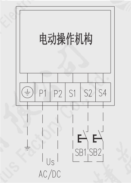
图 3-16 CD2型电动机操作机构接线图
