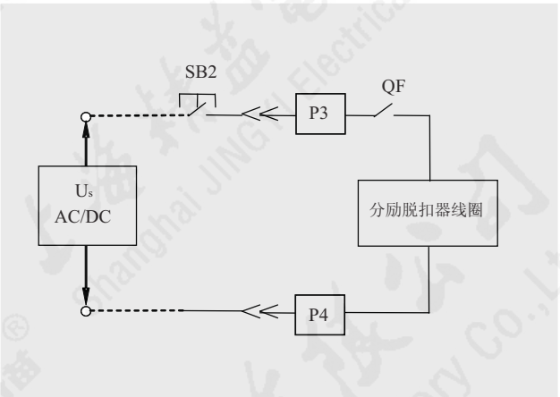
图 3-14 分励脱扣器二次回路接线图
