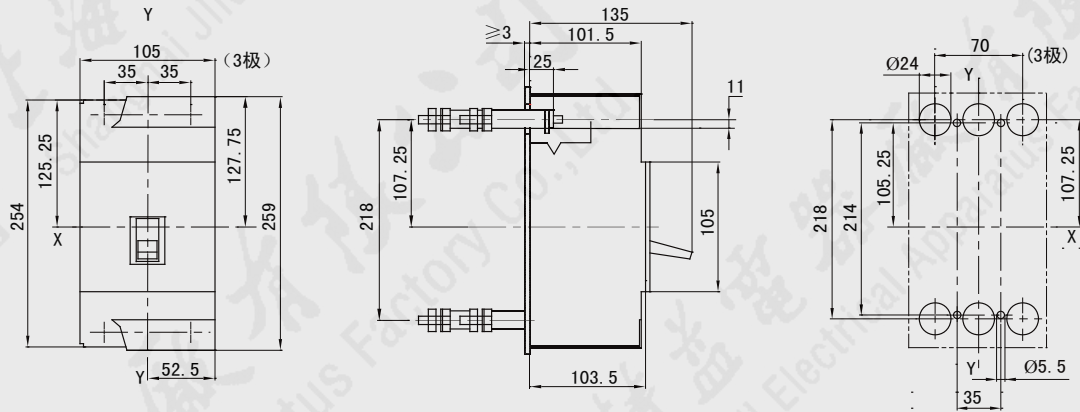
板后螺杆接线（电子式）
