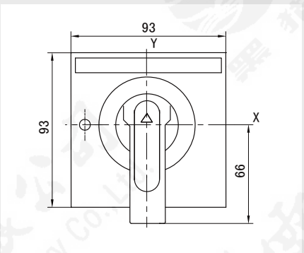
F-1 型 (用于HM3-63A~400A)
