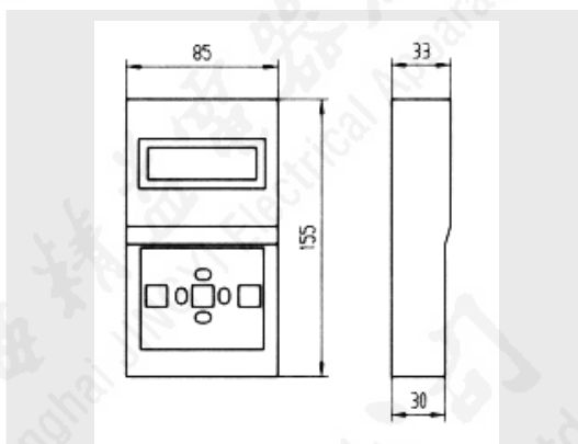
图2-9 ST型手持编程器外形尺寸图
