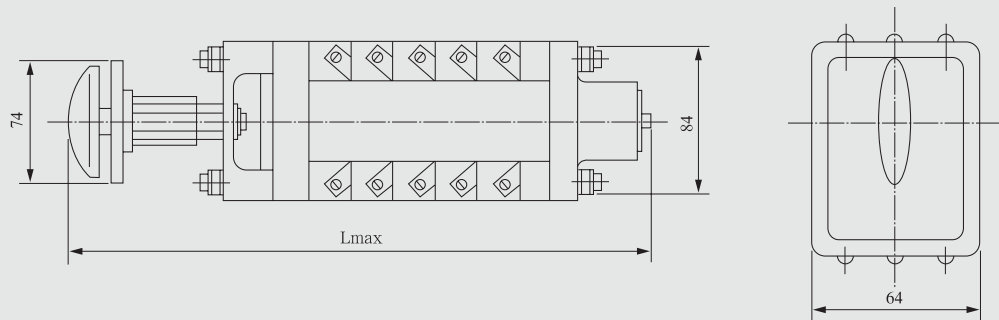
图1 自复(W)型: L_{max}=130+18n 其他型: L_{max}=141+18n 式中n-接触系统节数
