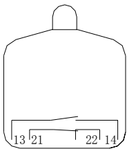
LXW20-11 (M) 型式
