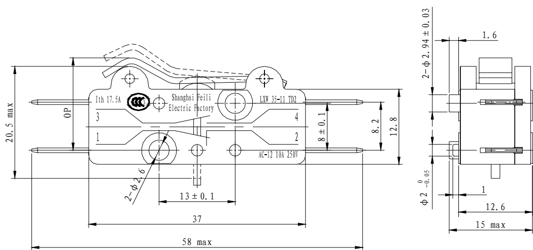
图12 LXW35-11TD2
