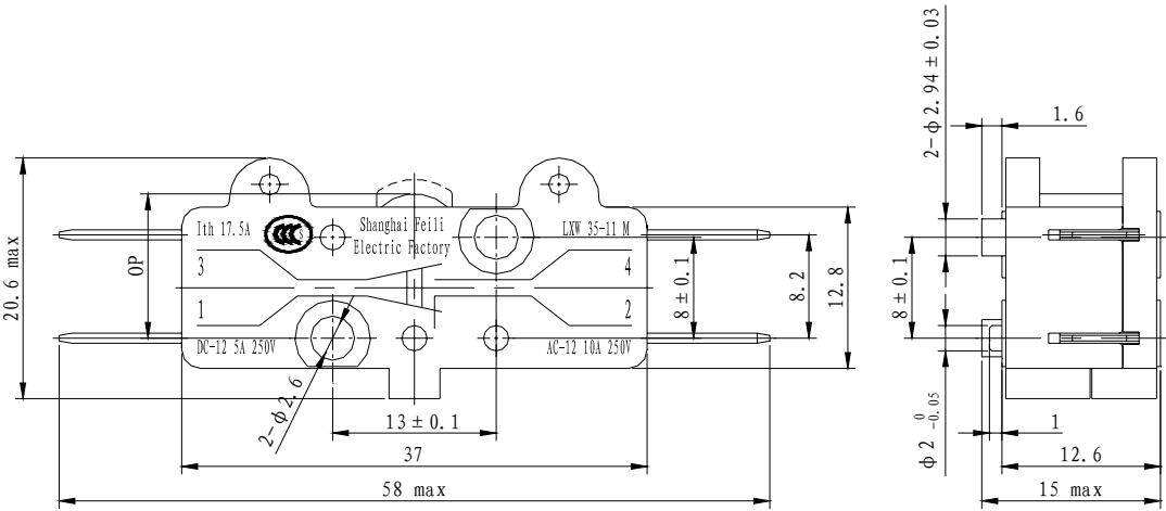
图1 LXW35-11M
