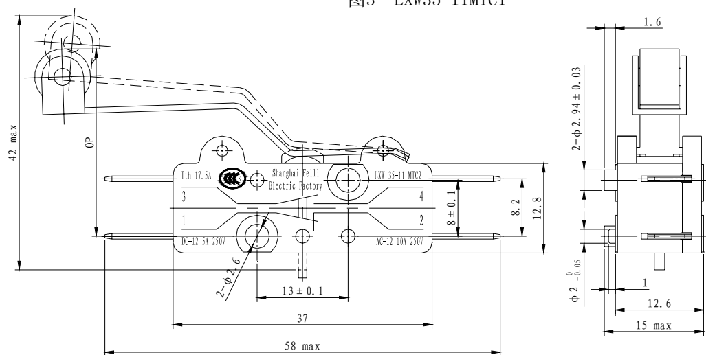
图4 LXW35-11MTC2
