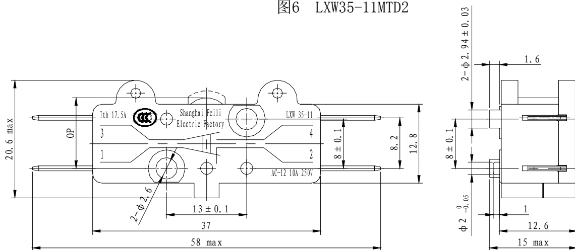
图7 LXW35-11
