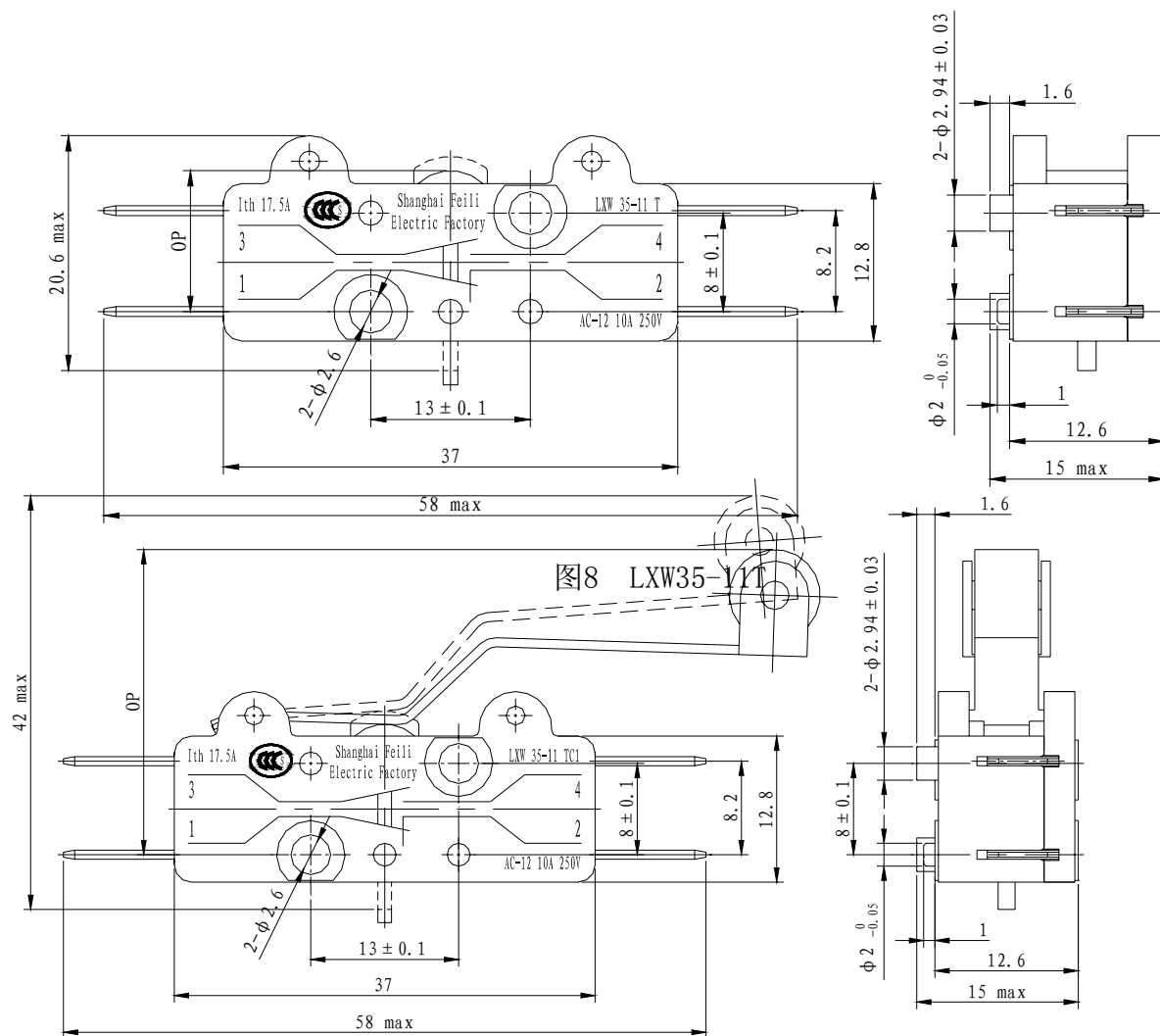
图9 LXW35-11TC1
