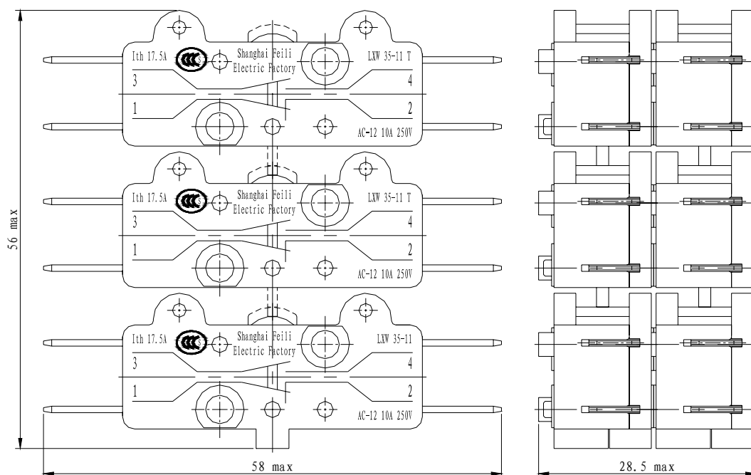
图16 六只开关组合成一组 Six switch combinations in together
