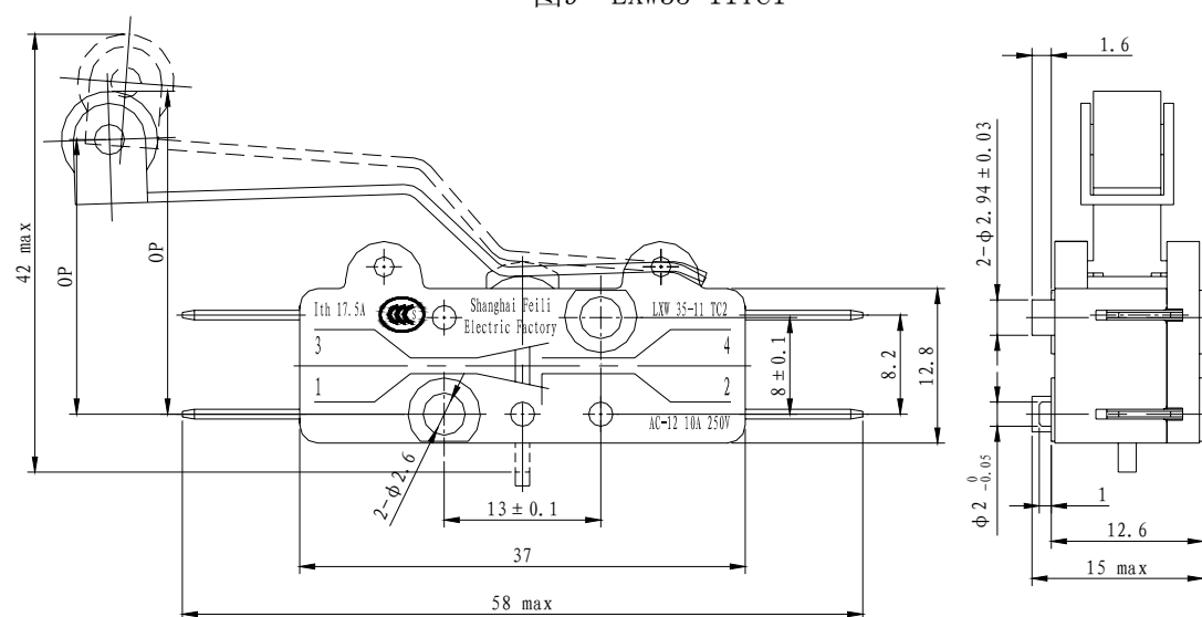
图10 LXW35-11TC2
