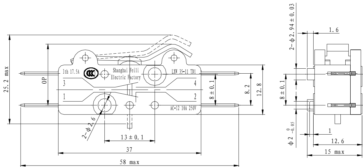
图11 LXW35-11TD1
