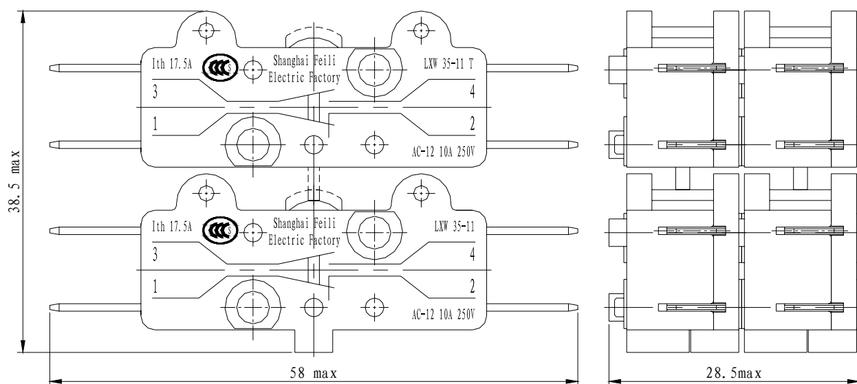
图15 四只开关组合成一组 Four switch combinations in together
