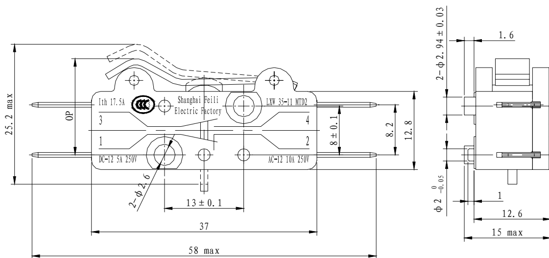
图6 LXW35-11MTD2
