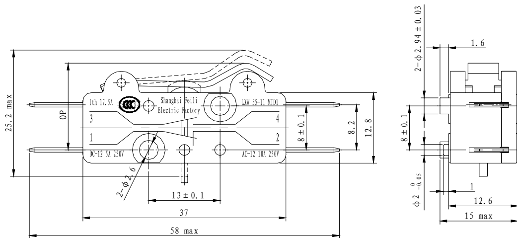
图5 LXW35-11MTD1
