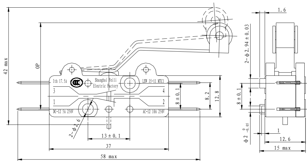
图2 LXW35-11MT
