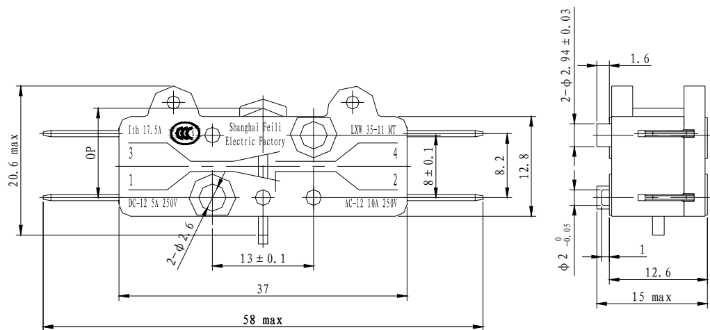
图2 LXW35-11MT
