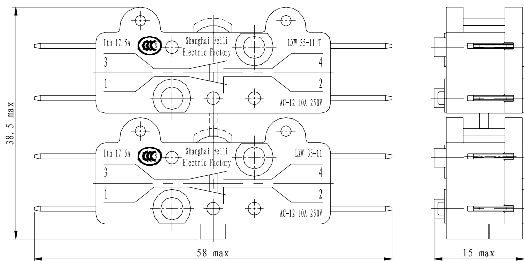
图13 二只开关组合成一组 Two switch combinations in together
