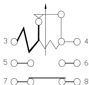
底视电路图
