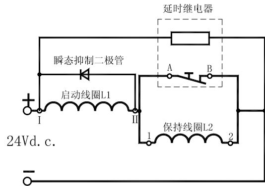
电磁铁电气原理图
