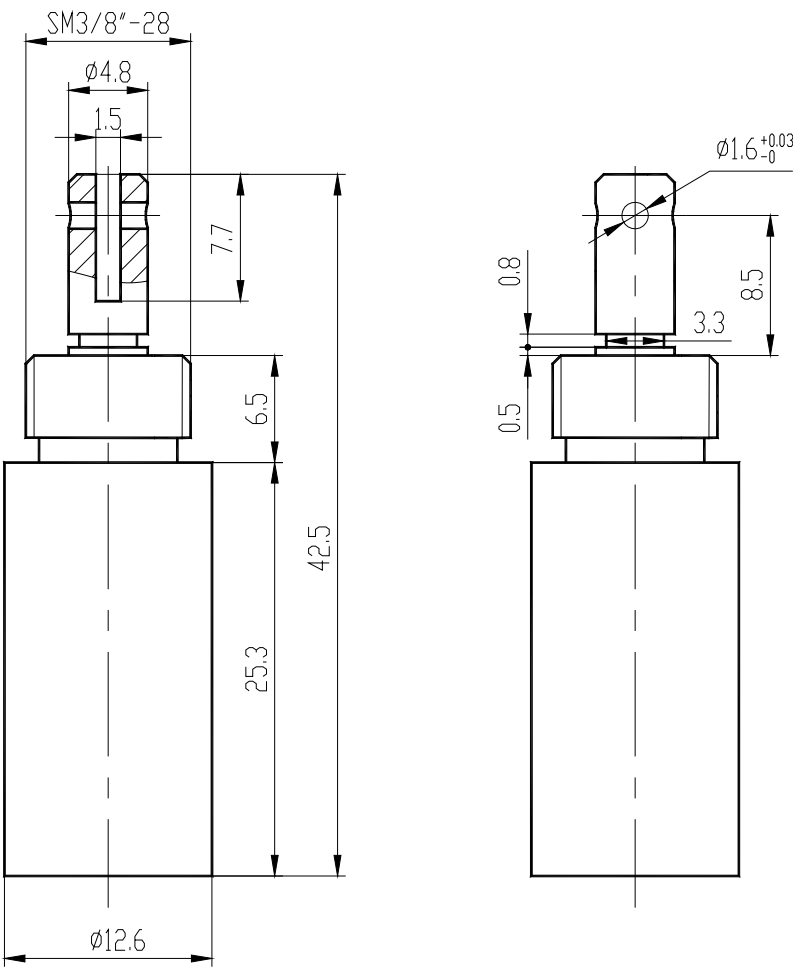
外形图及安装尺寸:
