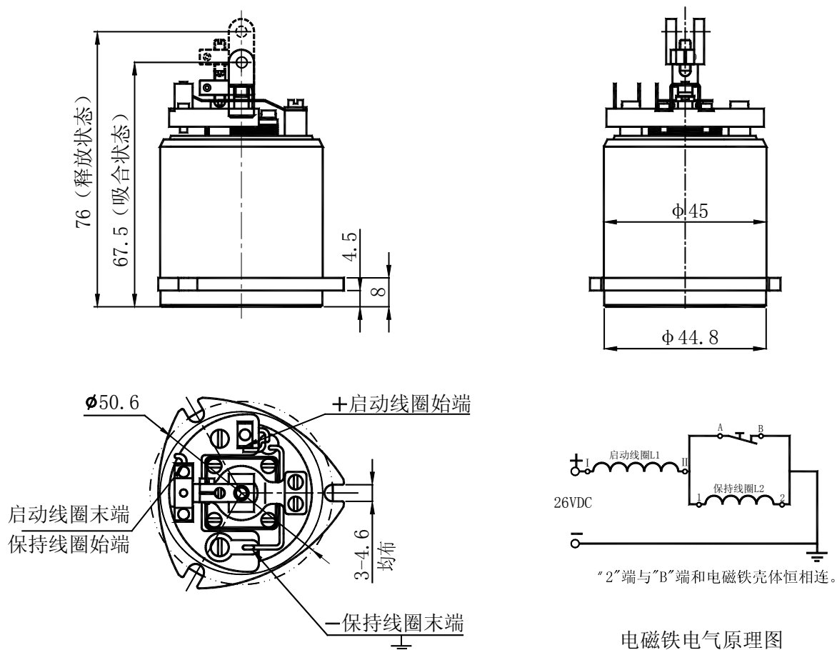
外形图及底视电路图
